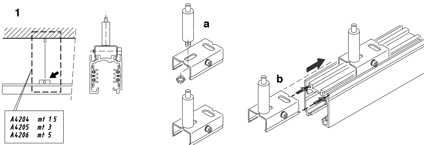
Fig. 1 Intestazione conduttori del binario Pic. 1 Recessing track conductors
