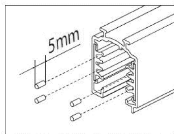
Fig. 2 Intestazione minima Pic. 2 Minimum recessing
