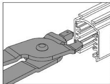
Fig. 1 Intestazione conduttori del binario Pic. 1 Recessing track conductors
